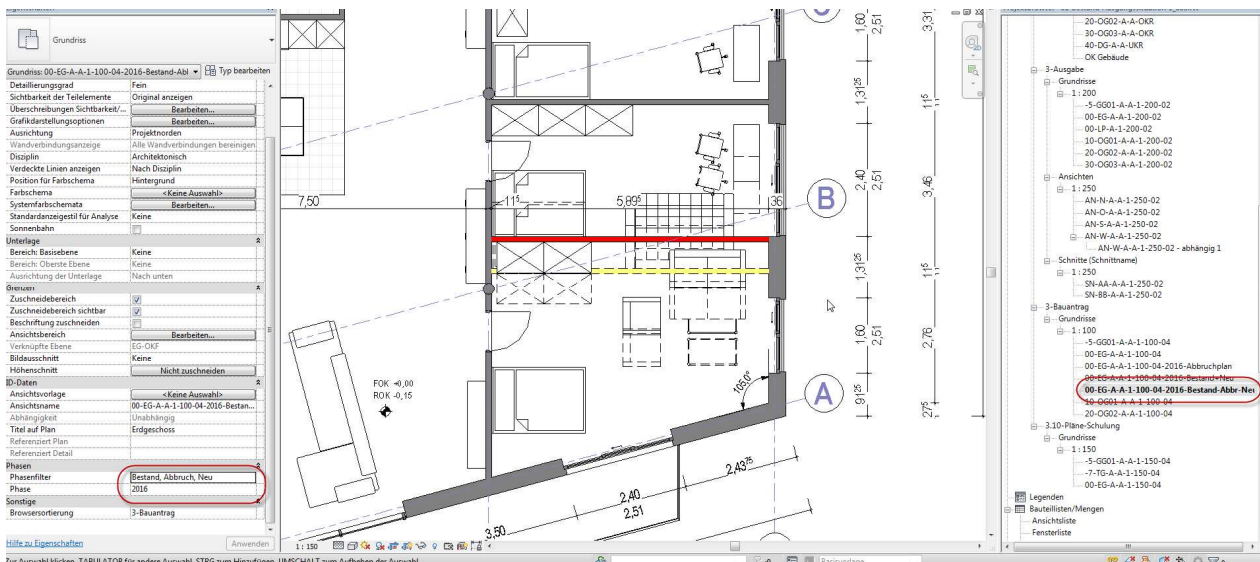
Abbildung 1.11-3: Plan Baugesuch – Phase 2016, Phasenfilter Bestand, Abbruch, Neu
