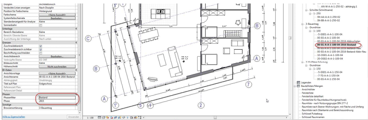
Abbildung 1.11-6: Plan Bestand vor Umbau – Phase 2015, Phasenfilter Bestand
