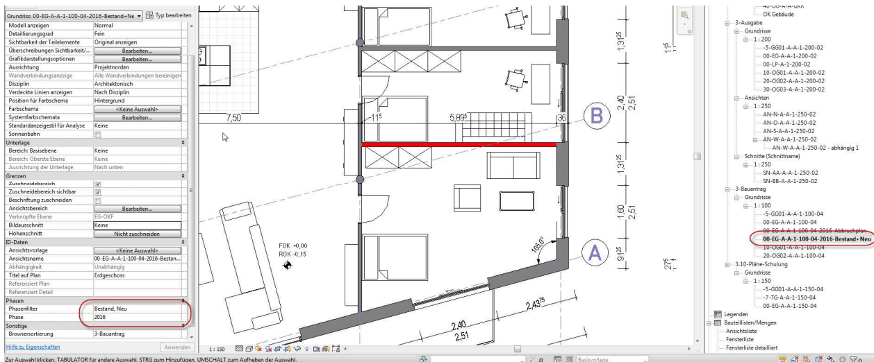
Abbildung 1.11-2: Plan Bestand und Neubau – Phase 2016, Phasenfilter Bestand, Neu
